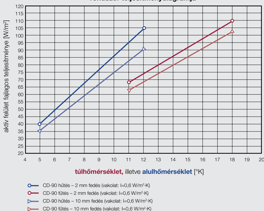
Wavin Tempower CW-90 felületfűtési és -hűtési rendszer teljesítménydiagramja
