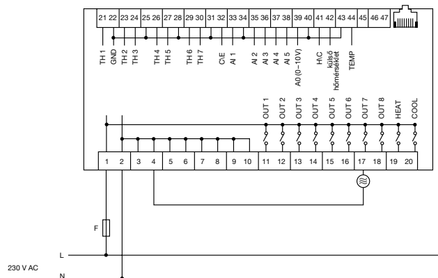
Légszárító bekötése a WTC-3-ba
