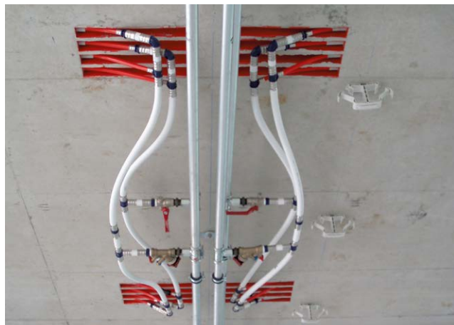
A födém a zsaluzat eltávolítása után a mennyezet alatt vezetett gyűjtővezetékkel és a bekötött CW-90 panelokkal
