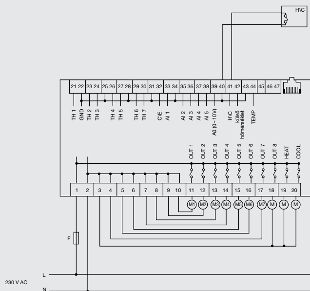
A WTC-3 bekötése analóg szobahőmérővel és külső fűtés/hűtés átkapcsolóval
