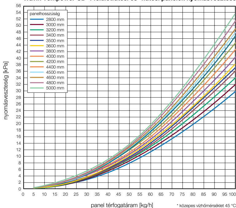
Wavin Tempower CD-4 felületfűtési és -hűtési panelek nyomásveszteség diagramja*
