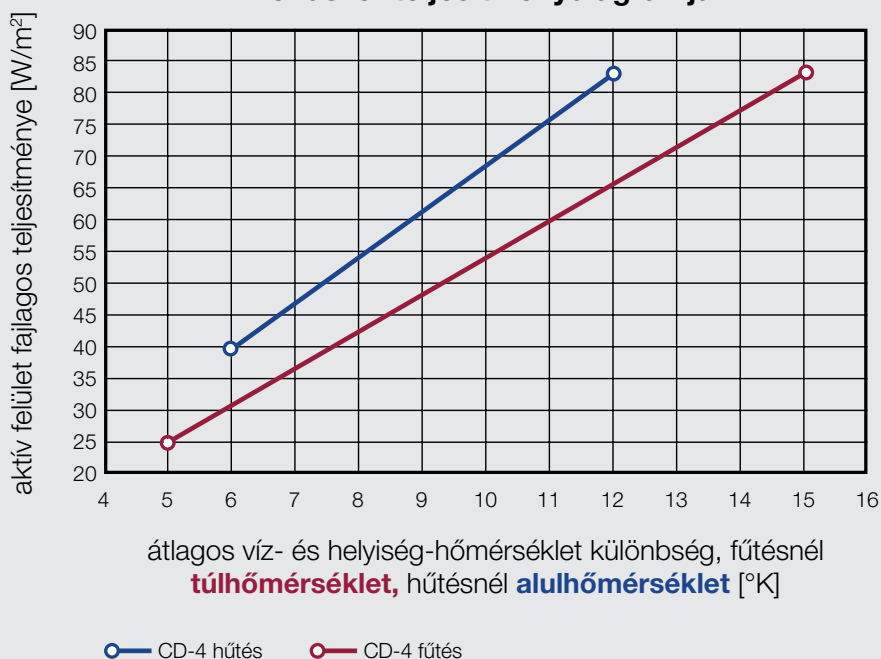
Wavin Tempower CD-4 felületfűtési és -hűtési rendszer teljesítménydiagramja
