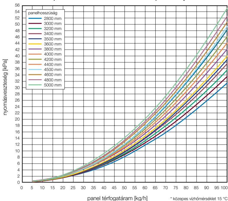
Nyomásveszteség diagram 15 °C-os közepes vízhőmérsékletnél (hűtés) Wavin Tempower CD-4 felületfűtési és -hűtési panelek nyomásveszteség diagram
