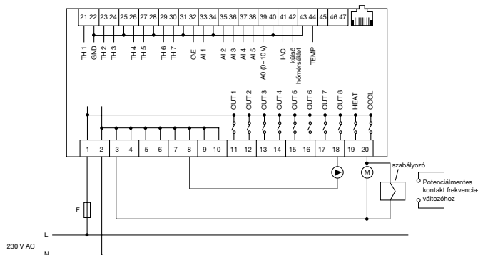
A WTC-3 szivattyúvezérlése potenciálmentes érintkezővel
