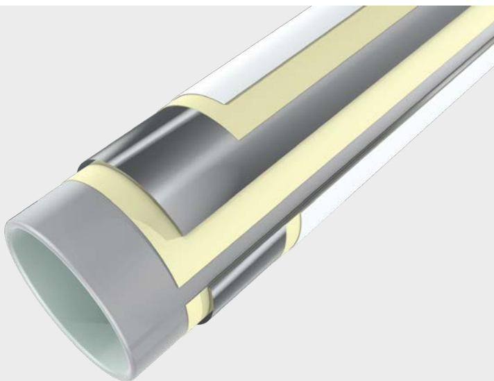
2. ábra: A Wavin PE-RT ötrétegű cső szerkezete
