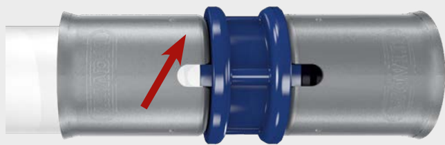
3. ábra: A rozsdamentes acél préshüvelyben található kémlelőnyíláson keresztül ellenőrizhető a cső ütközésig történő betolása
